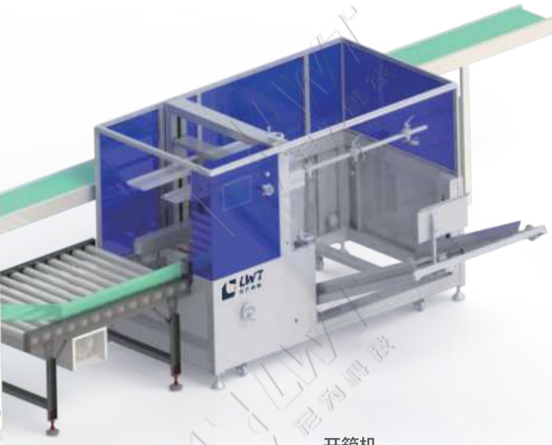
开箱机 Carton erector
