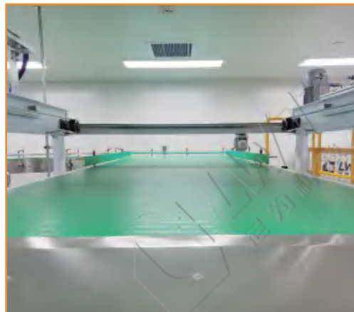
链板输送机 LW-DHP Chain plate conveyor LW-DHP
